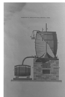
Rossiquel's apparatus for heating wine. ワインを暖めるためのロズイケ ル[ロシニョール]の装置
